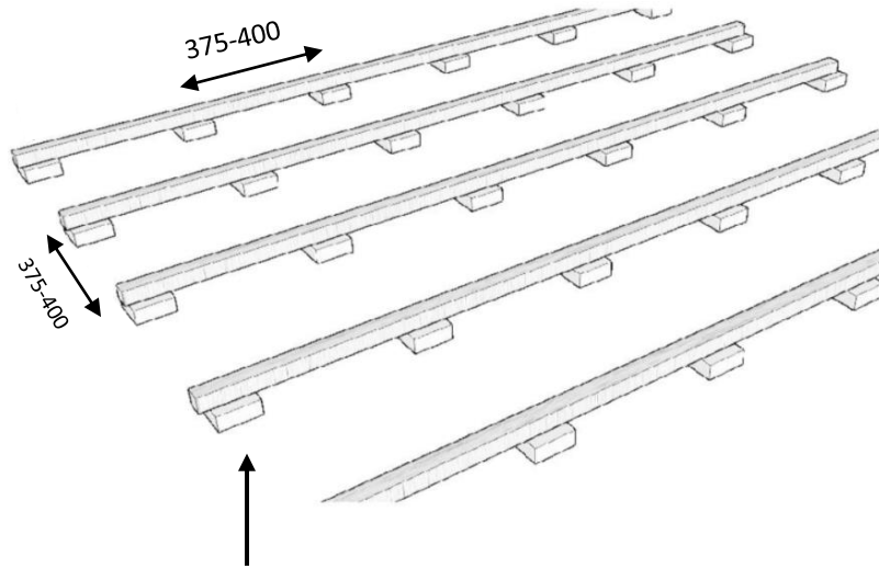
Zementfliesen unter den Balken.
